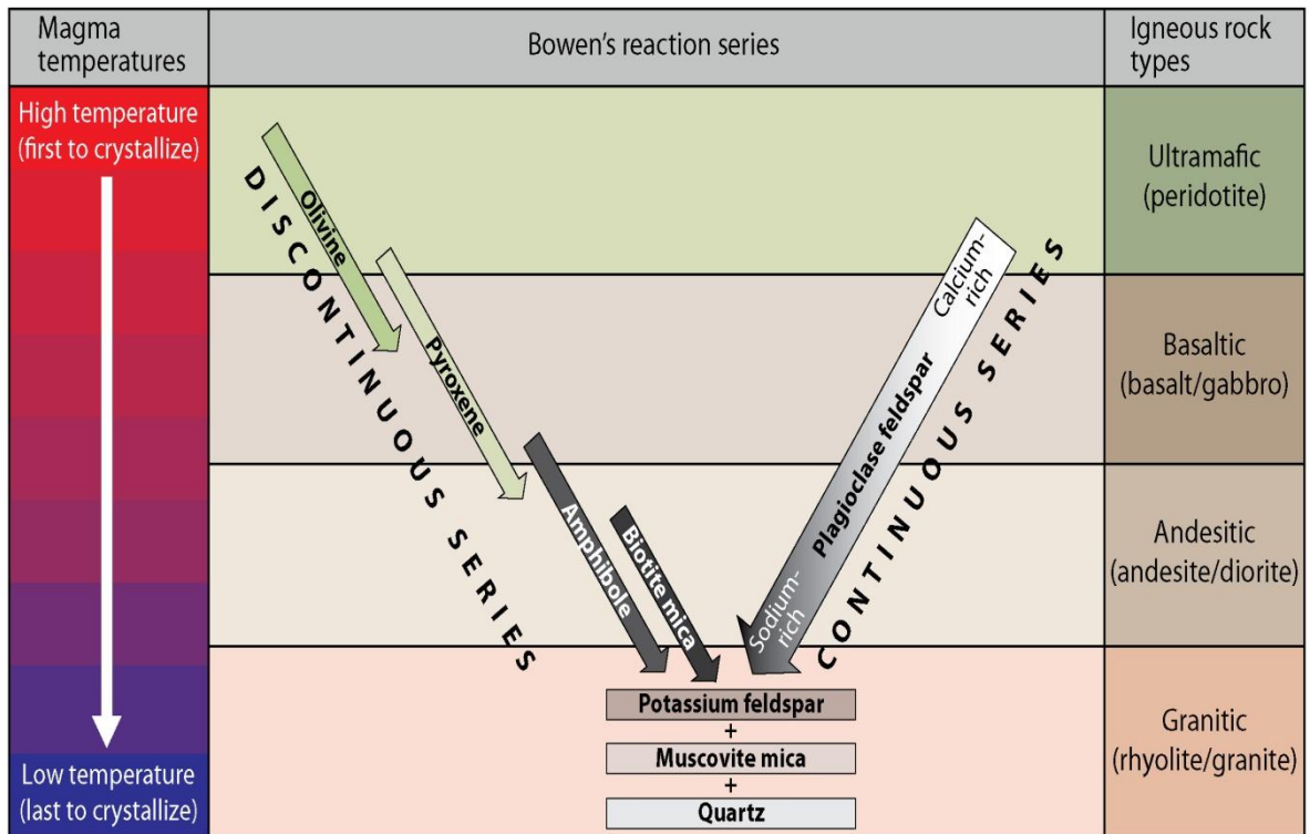
Figure 1 suites réactionnelles de Bowen
